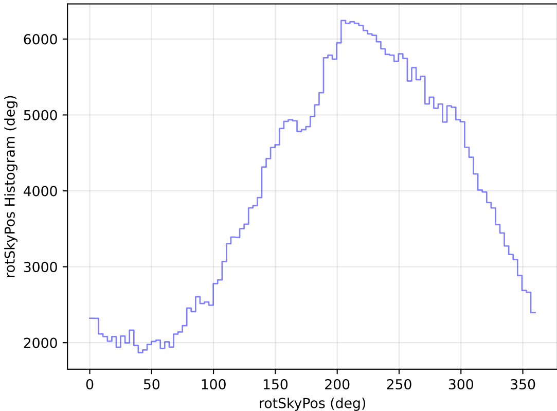
weather_cloudso2v3.4_10yrs All sky y band: rotSkyPos Histogram
