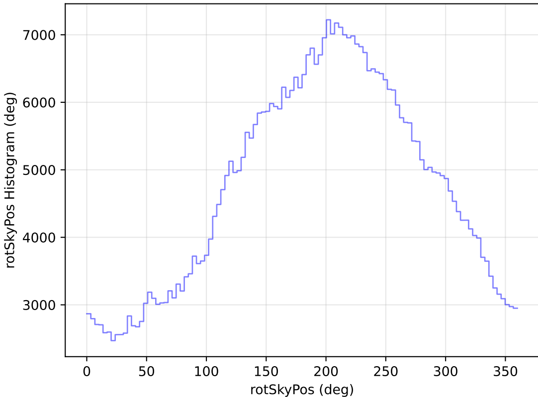
weather_cloudso2v3.4_10yrs All sky r band: rotSkyPos Histogram
