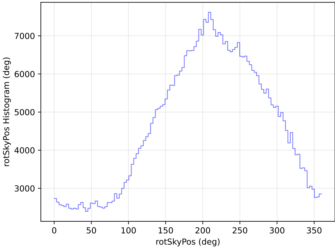
weather_cloudso2v3.4_10yrs All sky i band: rotSkyPos Histogram
