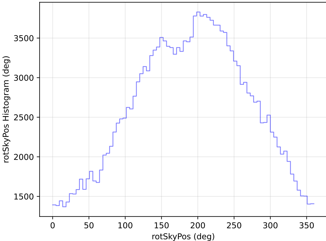
weather_cloudso2v3.4_10yrs All sky g band: rotSkyPos Histogram
