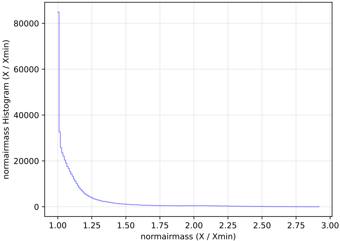
weather_cloudso2v3.4_10yrs WFD i band: normairmass Histogram
