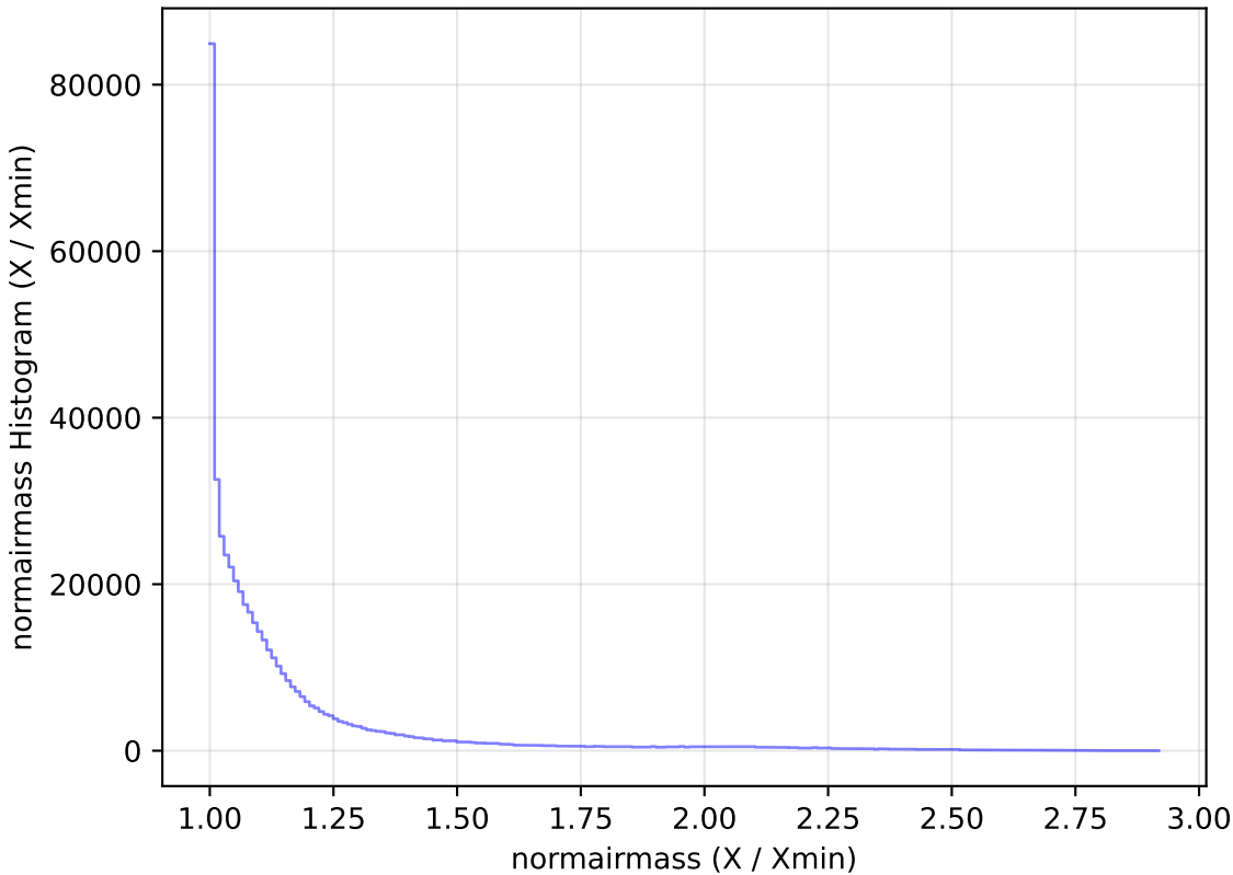
weather_cloudso2v3.4_10yrs All sky i band: normairmass Histogram
