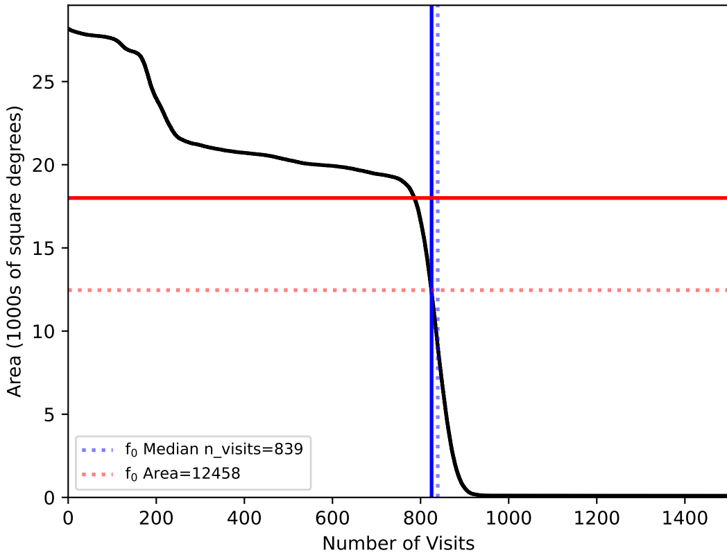
weather_cloudso2v3.4_10yrs All sky: f0
