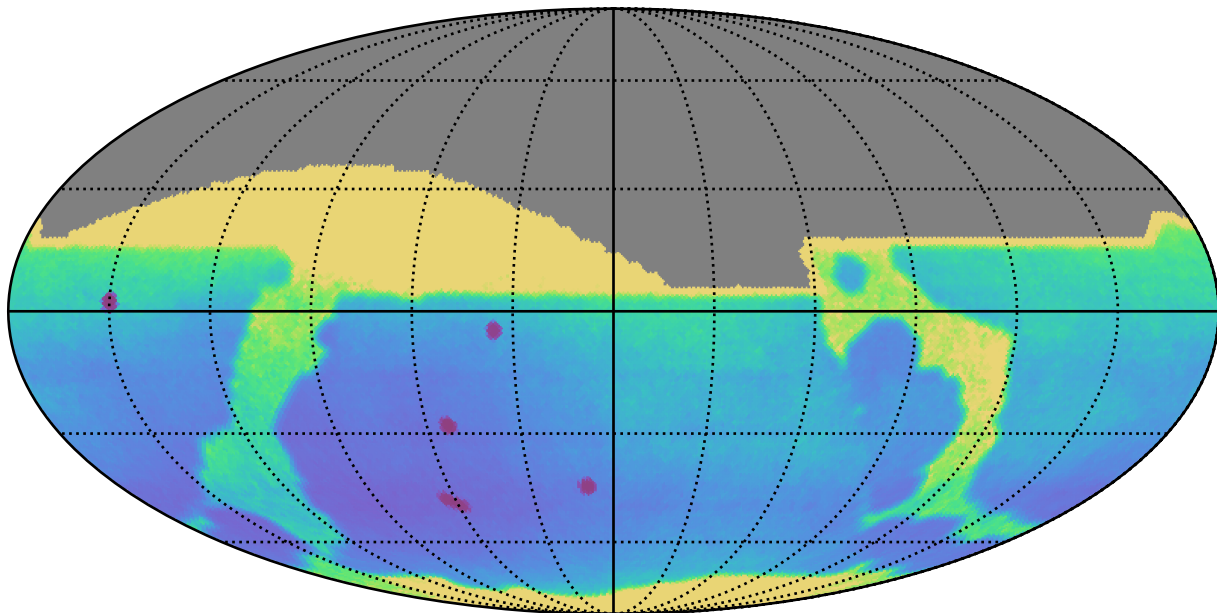
weather_cloudso2v3.4_10yrs All sky: Parallax Uncert @ 22.4
