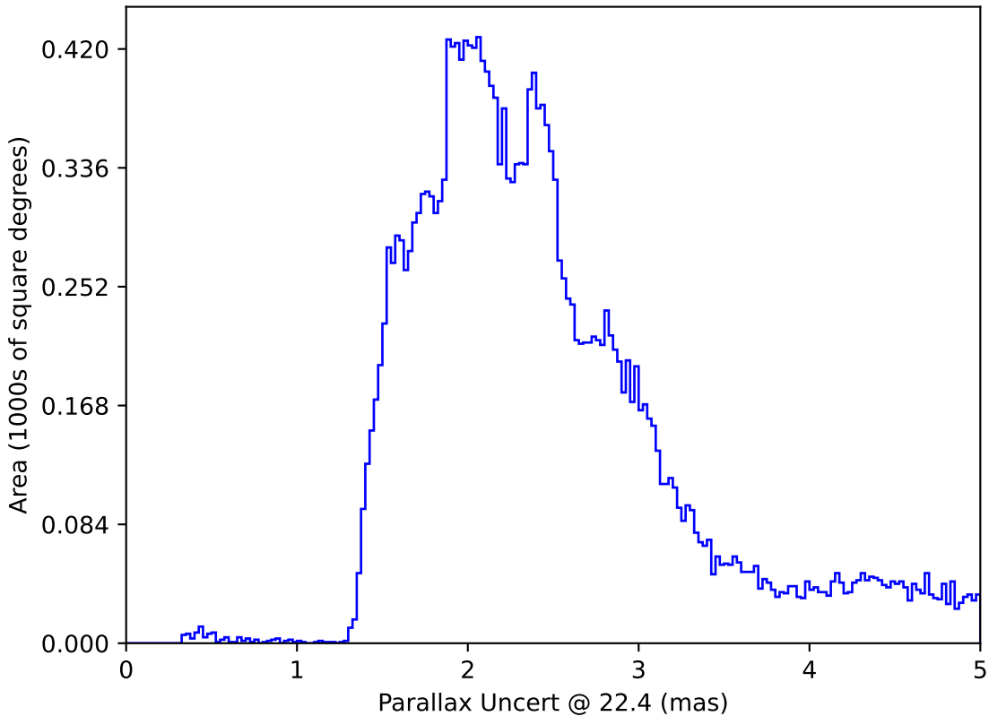
weather_cloudso2v3.4_10yrs All sky: Parallax Uncert @ 22.4
