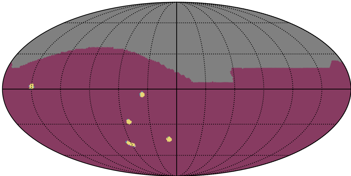
weather_cloudso2v3.4_10yrs All sky: NumberOfQuickRevisits
