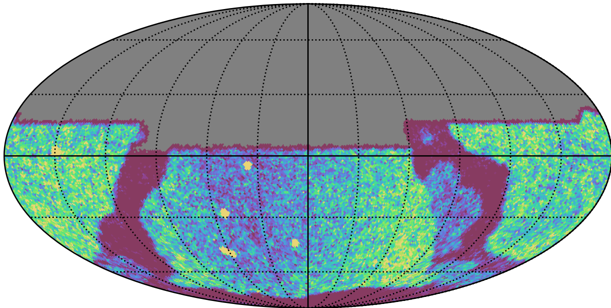
weather_cloudso2v3.4_10yrs Yr 1 y band: NVisits
