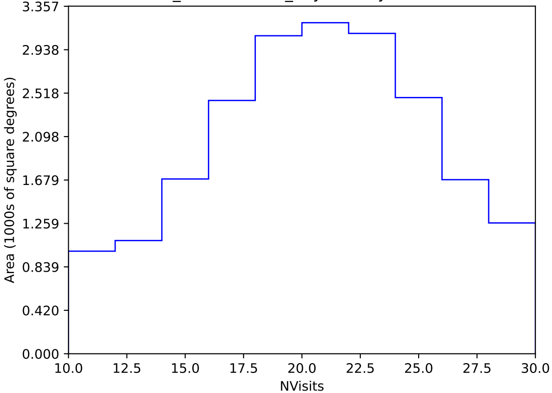
weather_cloudso2v3.4_10yrs Yr 1 y band: NVisits
