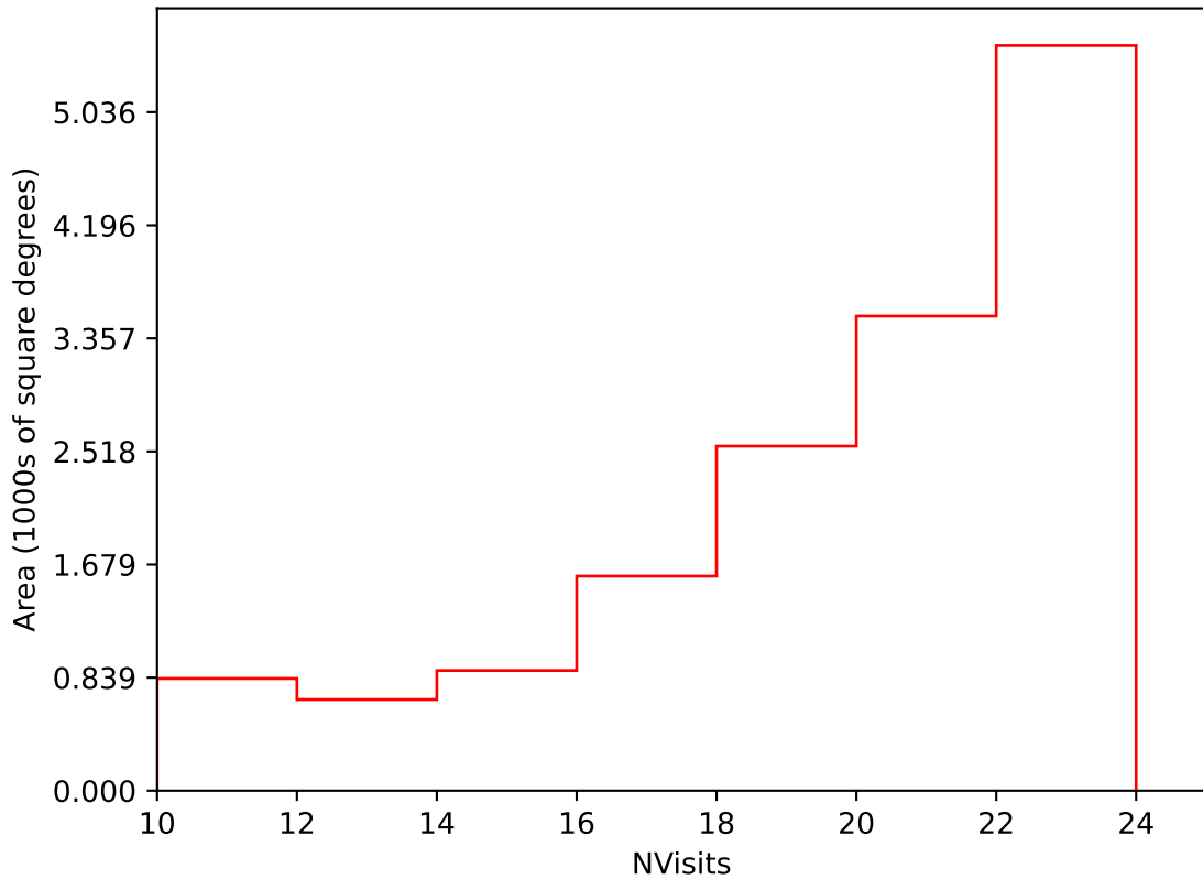
weather_cloudso2v3.4_10yrs Yr 1 i band: NVisits
