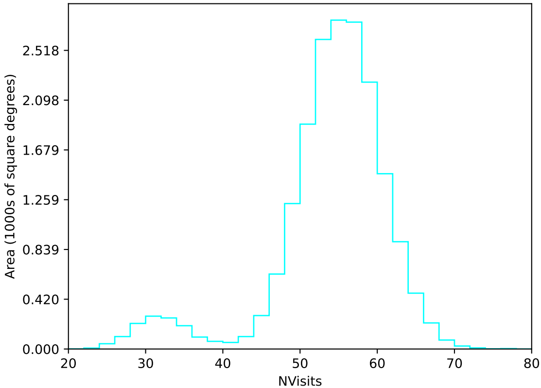
weather_cloudso2v3.4_10yrs WFD u band: NVisits
