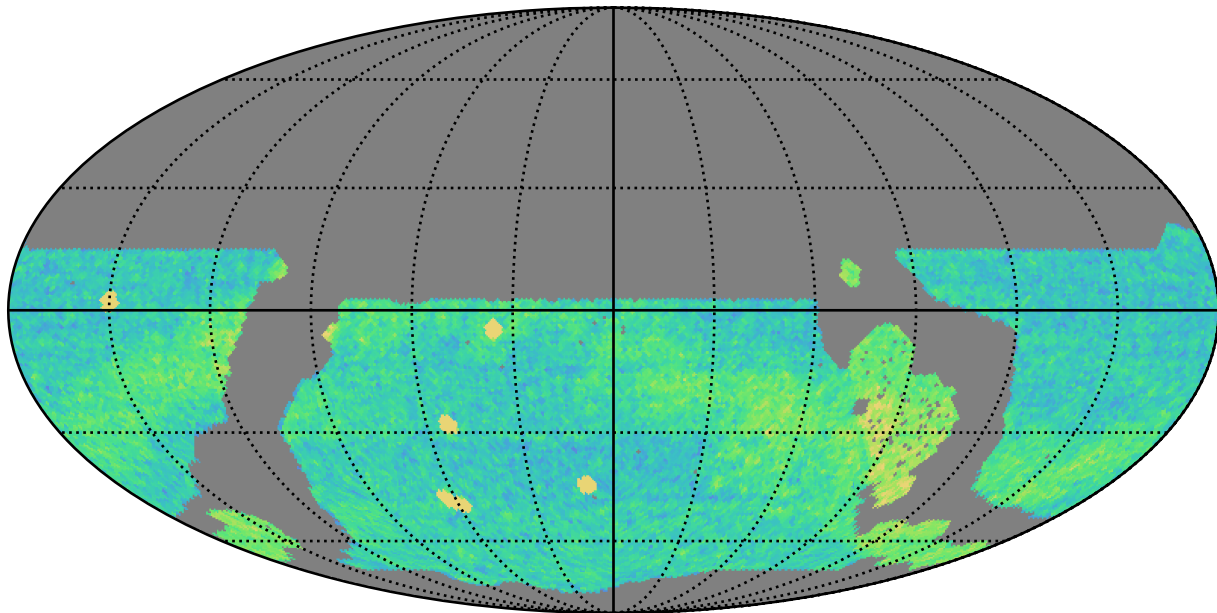
weather_cloudso2v3.4_10yrs WFD r band: NVisits
