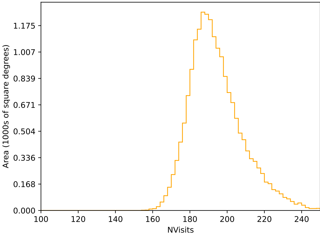
weather_cloudso2v3.4_10yrs WFD r band: NVisits
