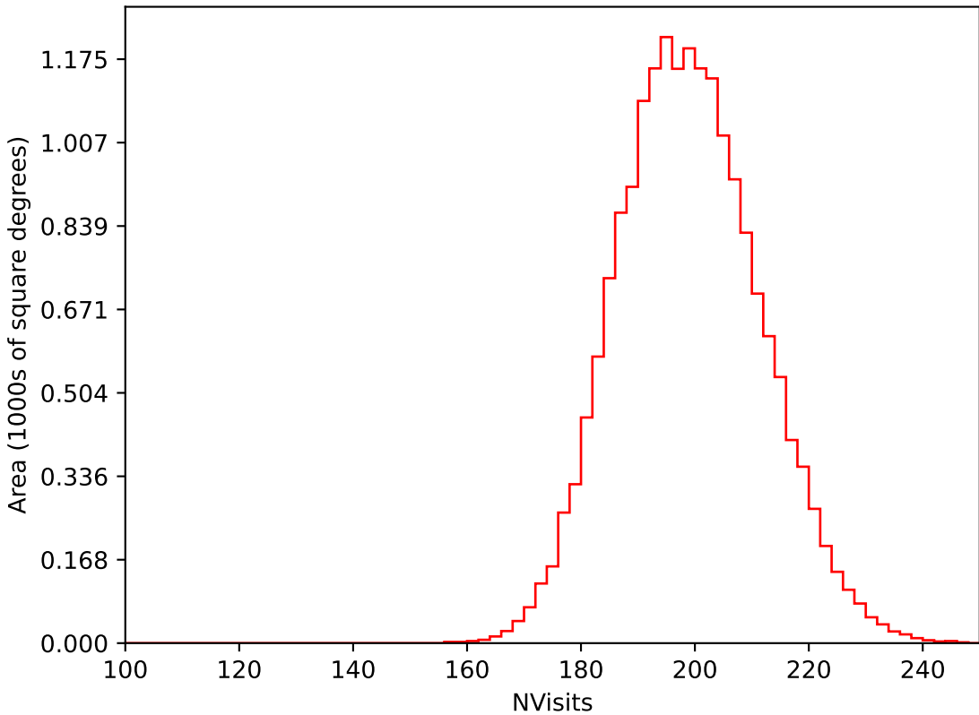
weather_cloudso2v3.4_10yrs WFD i band: NVisits
