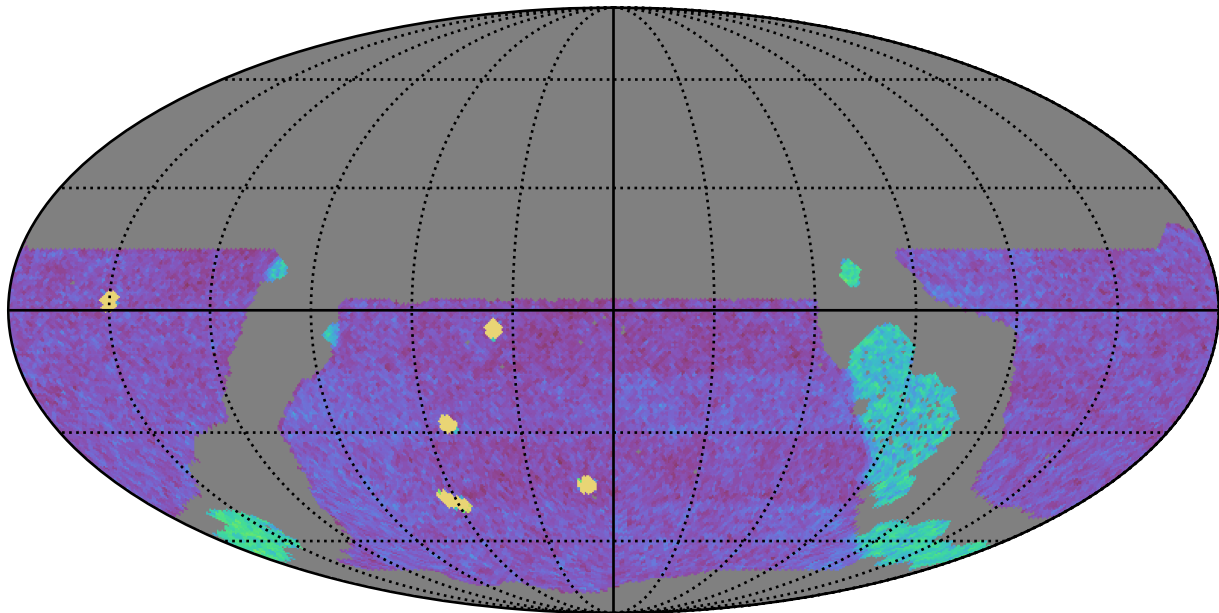
weather_cloudso2v3.4_10yrs WFD g band: NVisits
