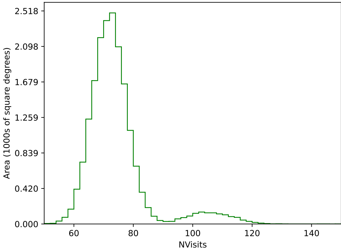
weather_cloudso2v3.4_10yrs WFD g band: NVisits
