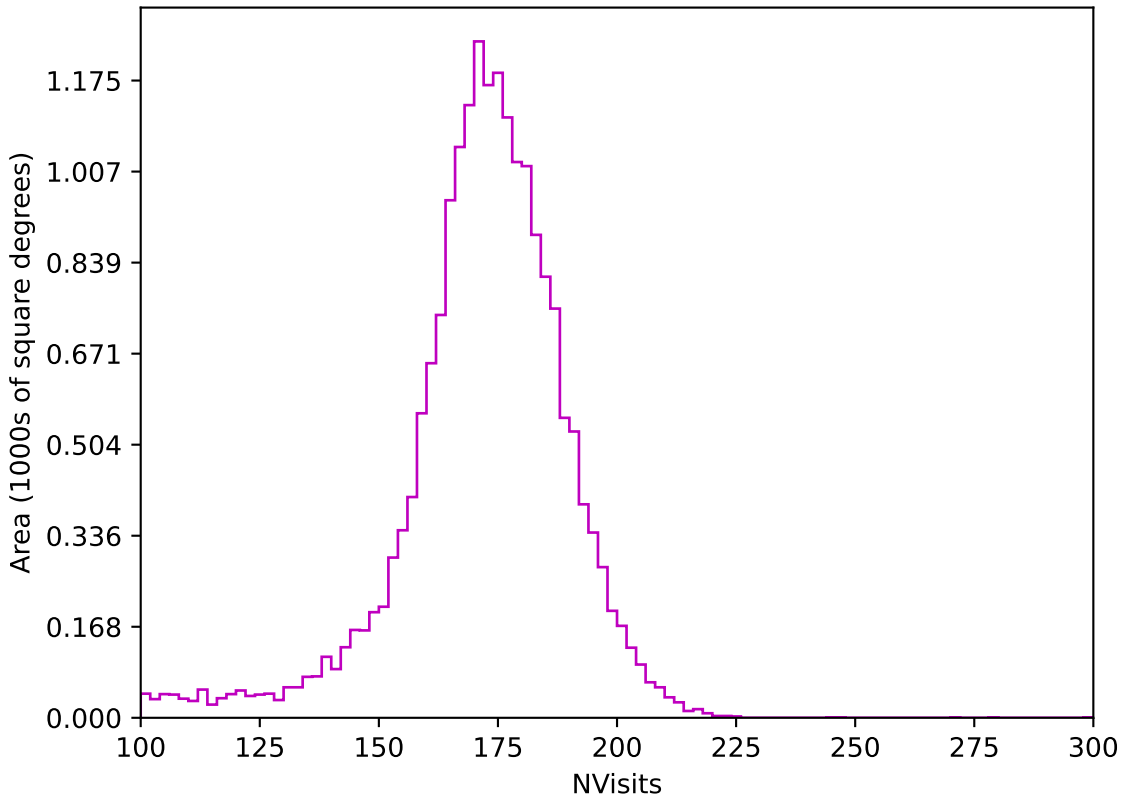
weather_cloudso2v3.4_10yrs All sky z band: NVisits
