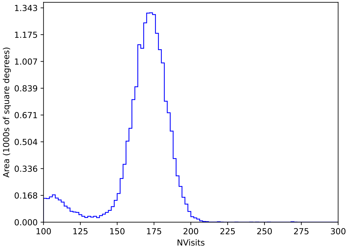
weather_cloudso2v3.4_10yrs All sky y band: NVisits
