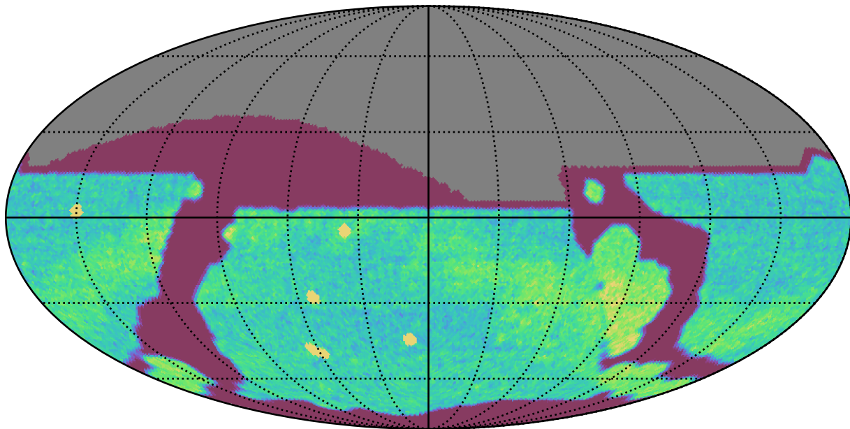
weather_cloudso2v3.4_10yrs All sky r band: NVisits
