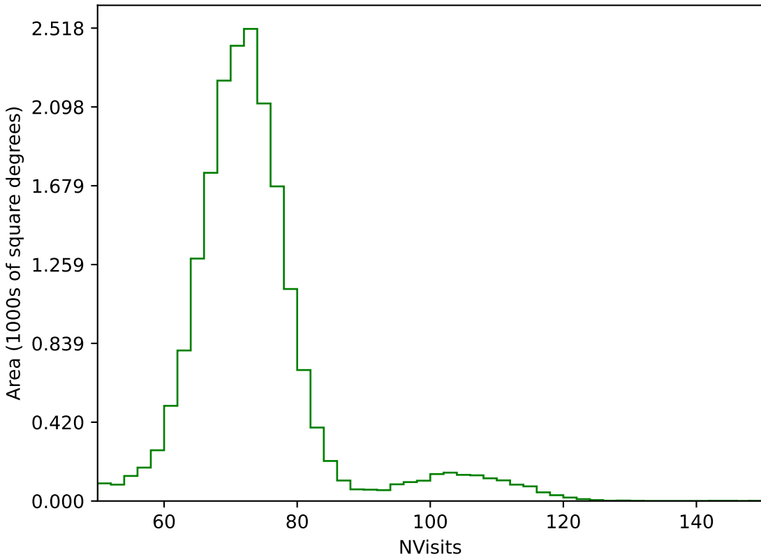
weather_cloudso2v3.4_10yrs All sky g band: NVisits
