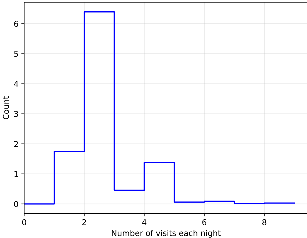
1e6 weather_cloudso2v3.4_10yrs All sky: NVisitsPerNight
