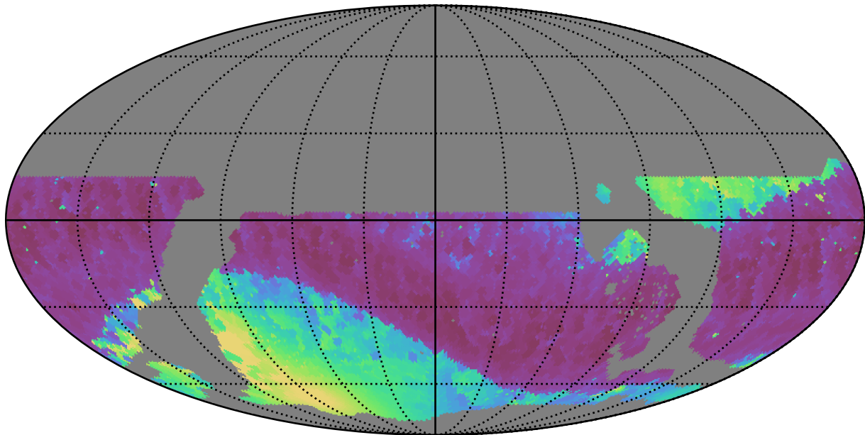
weather_cloudso2v3.4_10yrs WFD z band: Min solarElong
