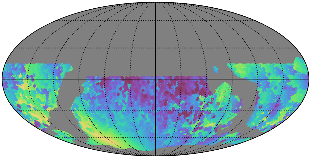
weather_cloudso2v3.4_10yrs WFD y band: Min solarElong
