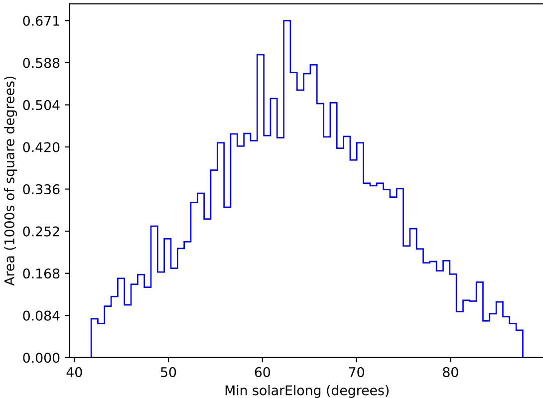
weather_cloudso2v3.4_10yrs WFD y band: Min solarElong
