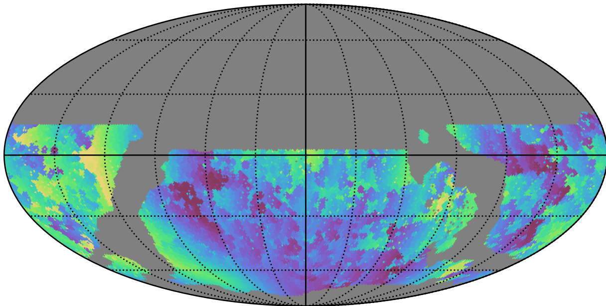
weather_cloudso2v3.4_10yrs WFD u band: Min solarElong
