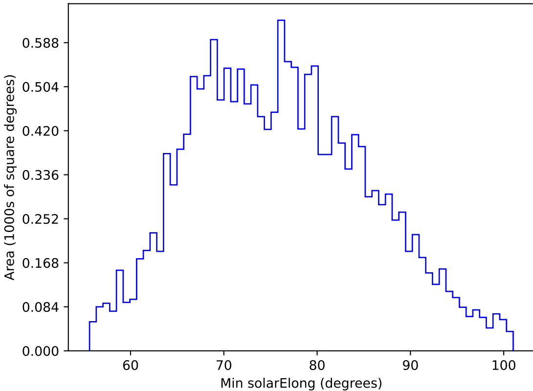
weather_cloudso2v3.4_10yrs WFD u band: Min solarElong
