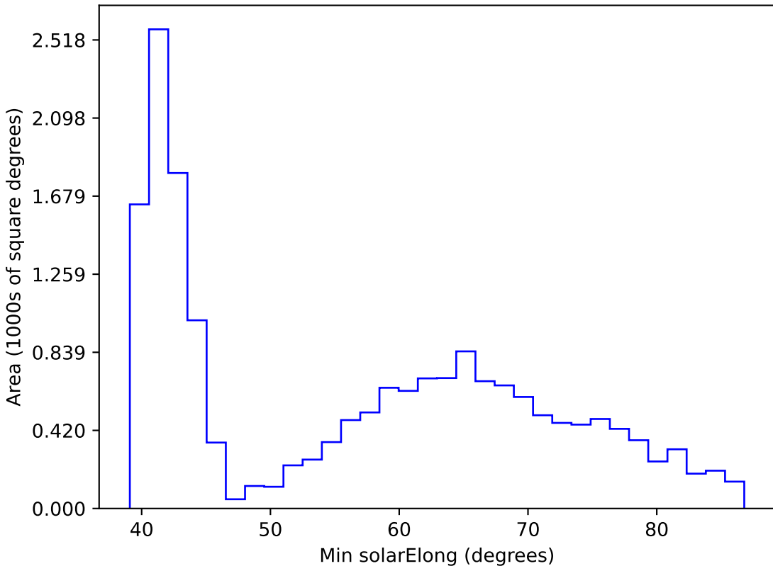
weather_cloudso2v3.4_10yrs WFD r band: Min solarElong
