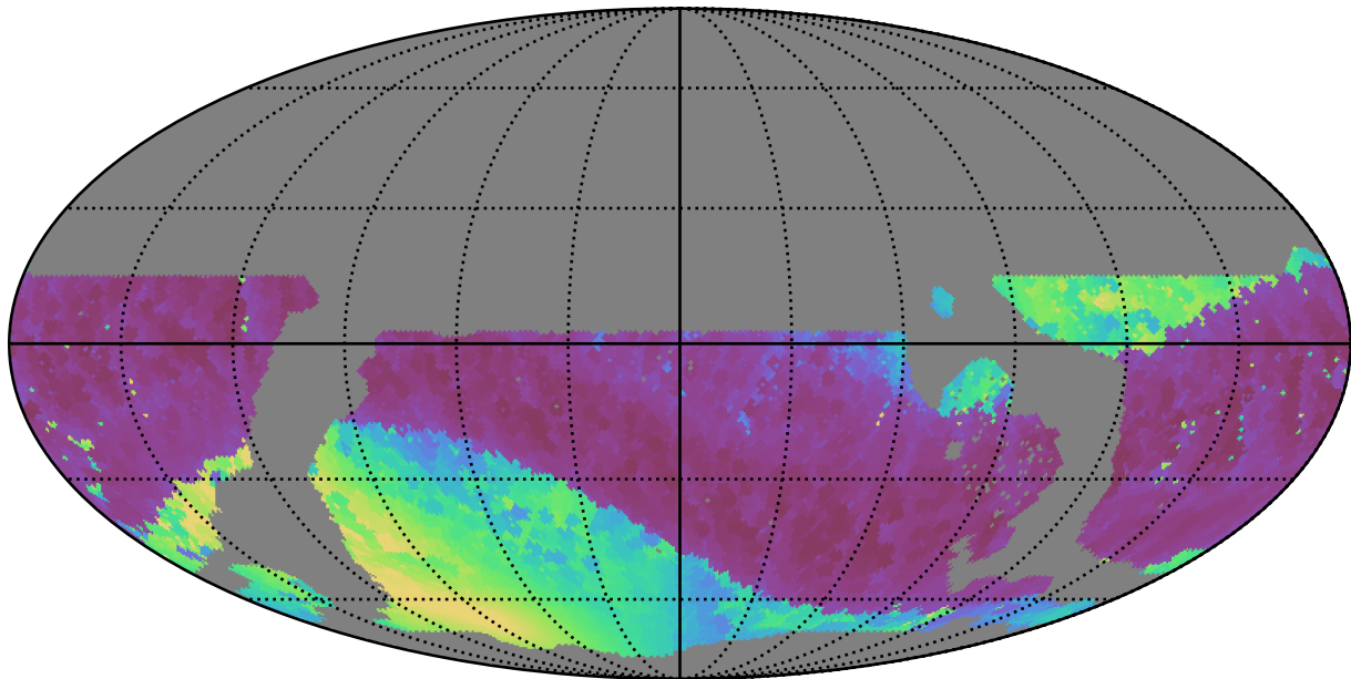
weather_cloudso2v3.4_10yrs WFD i band: Min solarElong
