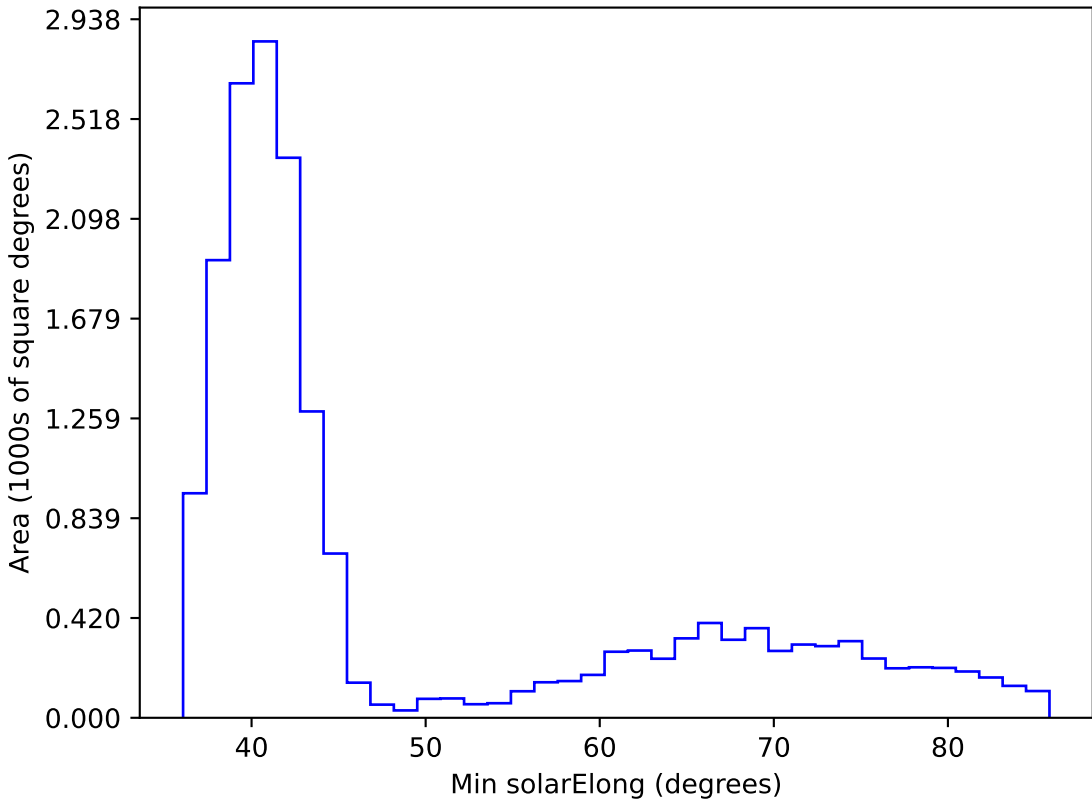
weather_cloudso2v3.4_10yrs WFD i band: Min solarElong
