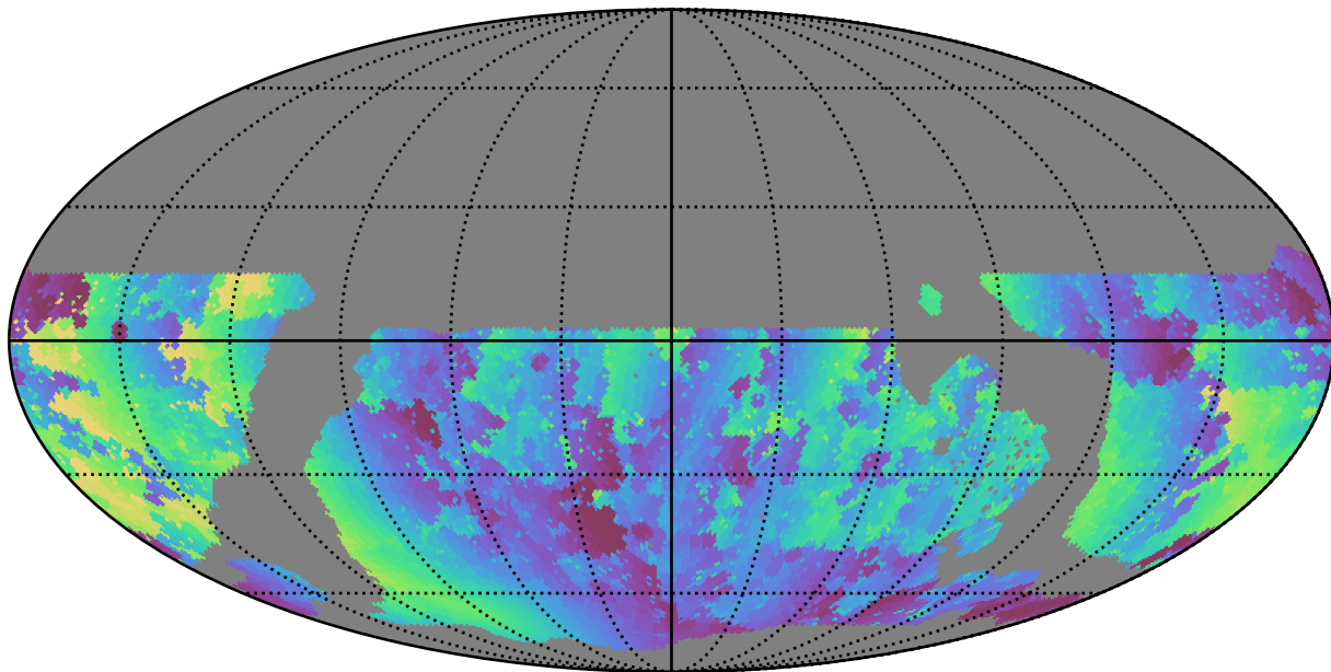
weather_cloudso2v3.4_10yrs WFD g band: Min solarElong
