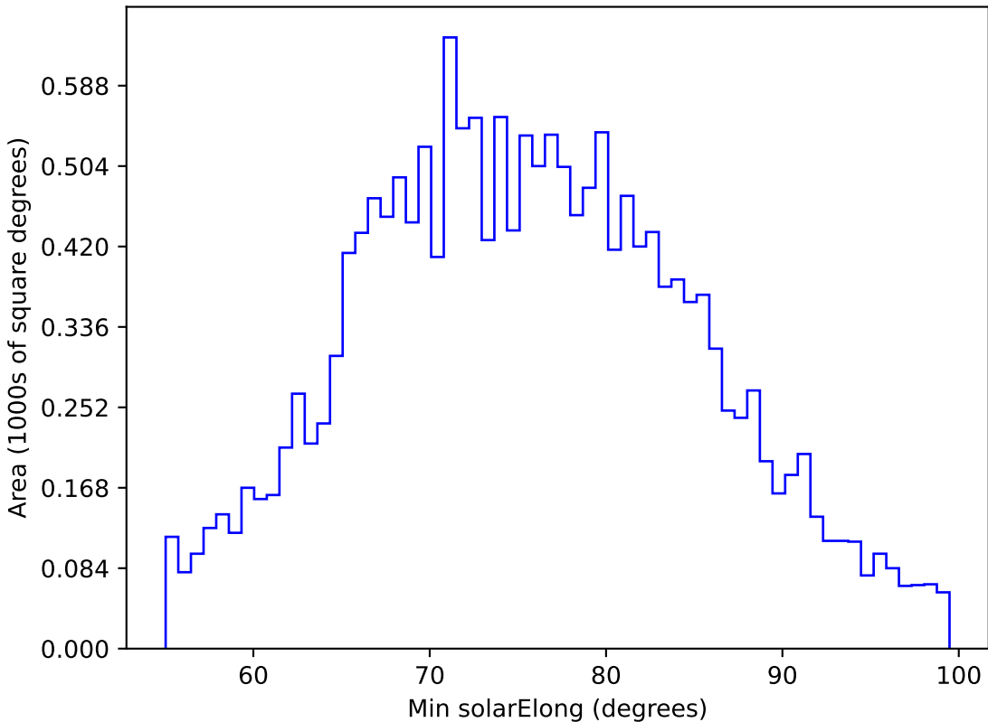
weather_cloudso2v3.4_10yrs WFD g band: Min solarElong
