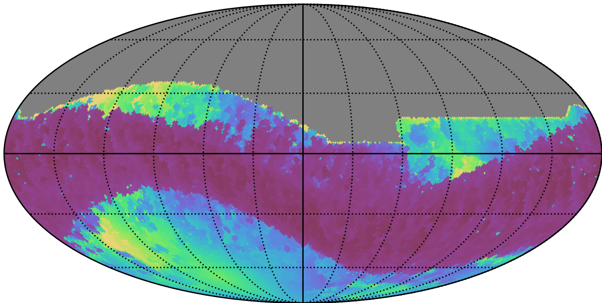
weather_cloudso2v3.4_10yrs All sky z band: Min solarElong
