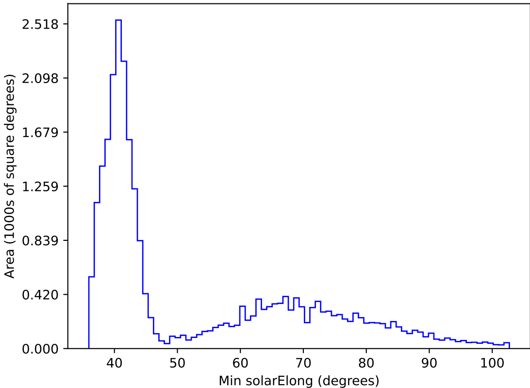
weather_cloudso2v3.4_10yrs All sky z band: Min solarElong
