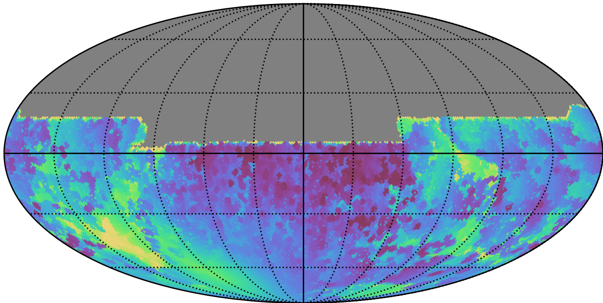
weather_cloudso2v3.4_10yrs All sky y band: Min solarElong
