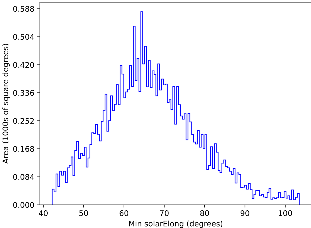
weather_cloudso2v3.4_10yrs All sky y band: Min solarElong
