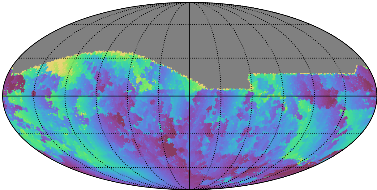
weather_cloudso2v3.4_10yrs All sky g band: Min solarElong
