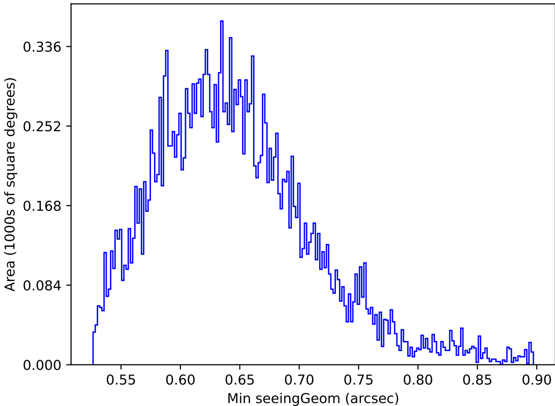
weather_cloudso2v3.4_10yrs Yr 1 y band: Min seeingGeom
