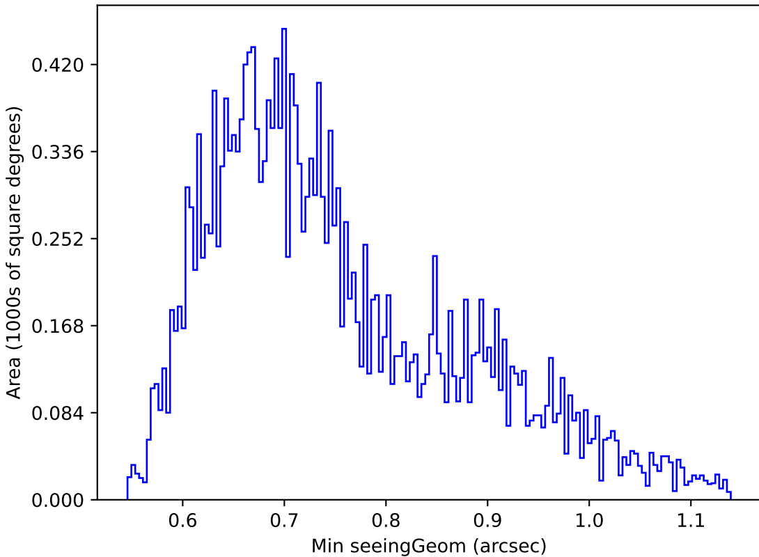
weather_cloudso2v3.4_10yrs Yr 1 u band: Min seeingGeom
