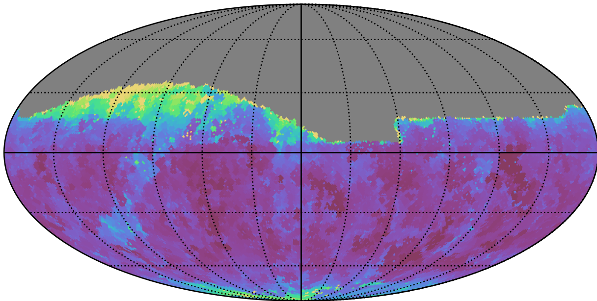
weather_cloudso2v3.4_10yrs Yr 1 i band: Min seeingGeom
