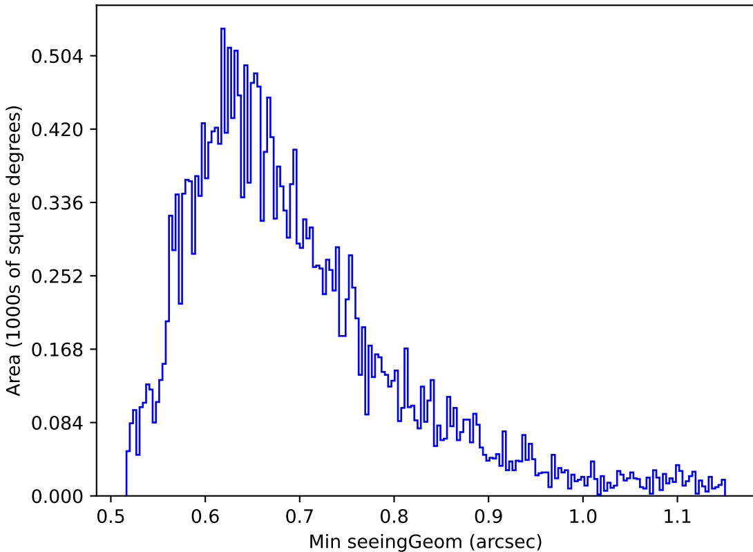
weather_cloudso2v3.4_10yrs Yr 1 g band: Min seeingGeom
