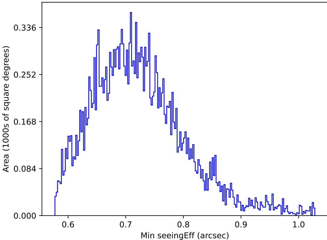
weather_cloudso2v3.4_10yrs Yr 1 y band: Min seeingEff
