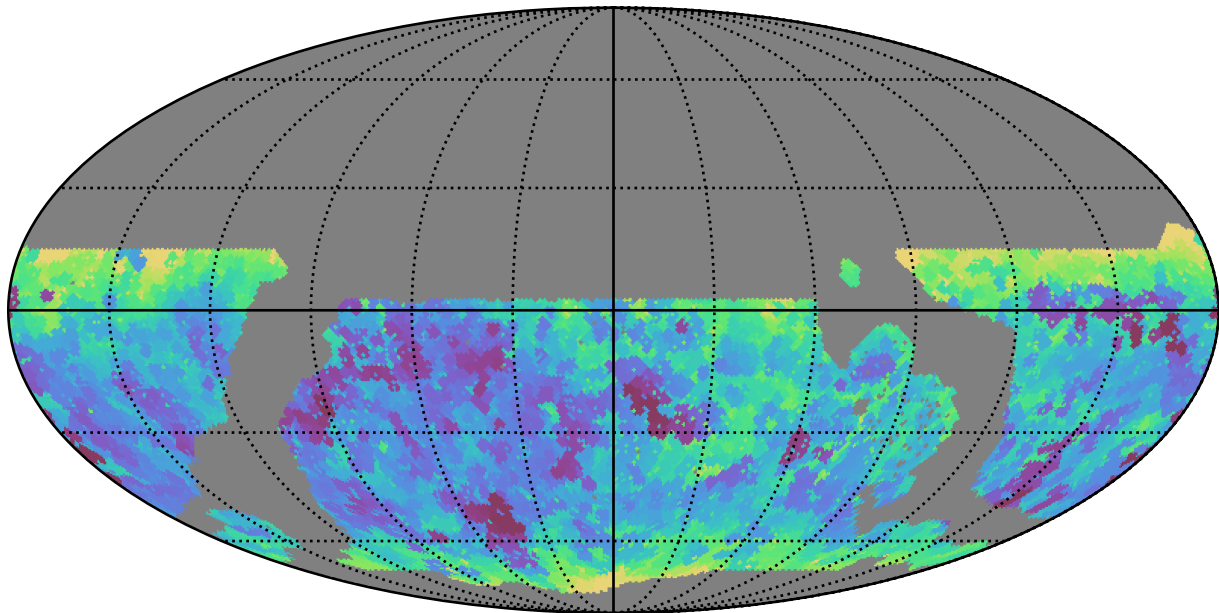
weather_cloudso2v3.4_10yrs WFD z band: Min seeingEff
