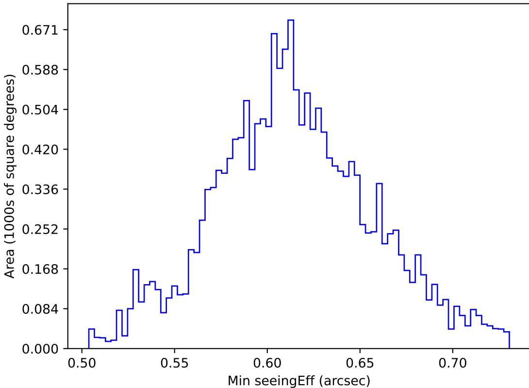
weather_cloudso2v3.4_10yrs WFD z band: Min seeingEff
