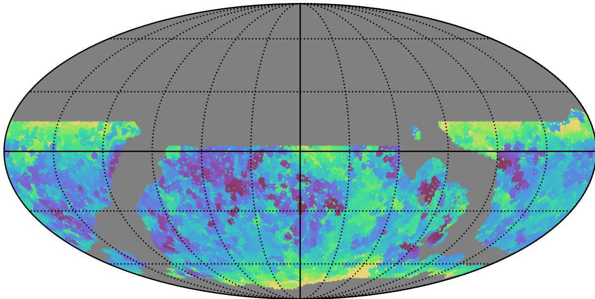
weather_cloudso2v3.4_10yrs WFD i band: Min seeingEff
