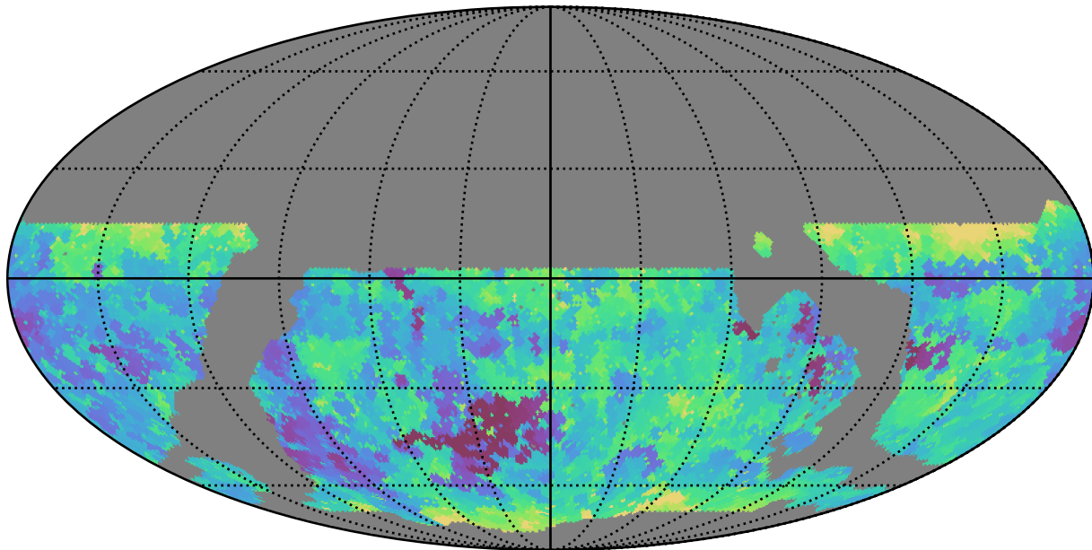
weather_cloudso2v3.4_10yrs WFD g band: Min seeingEff
