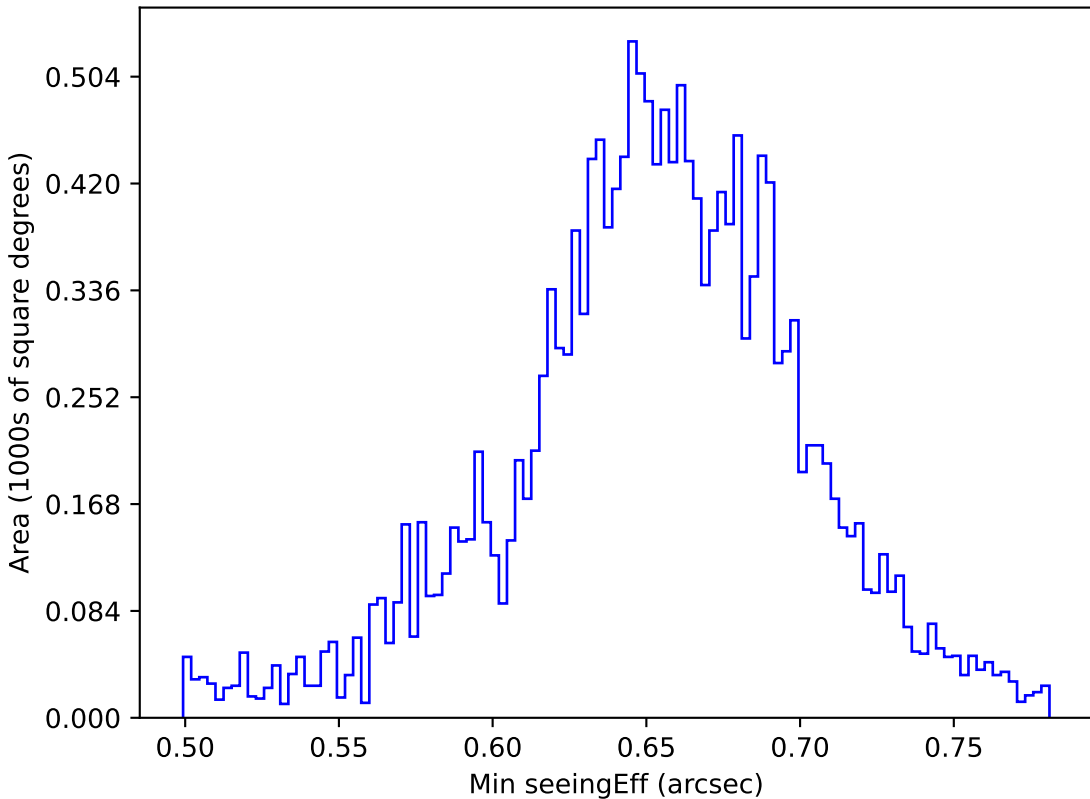
weather_cloudso2v3.4_10yrs WFD g band: Min seeingEff
