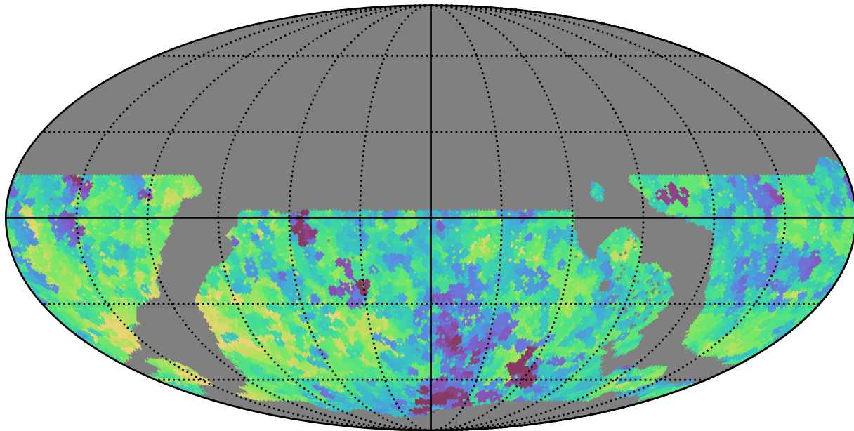
weather_cloudso2v3.4_10yrs WFD z band: Min saturation_mag
